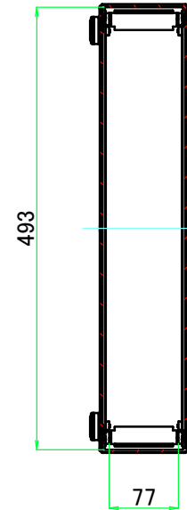
B-B ( 1 : 7.5 )
